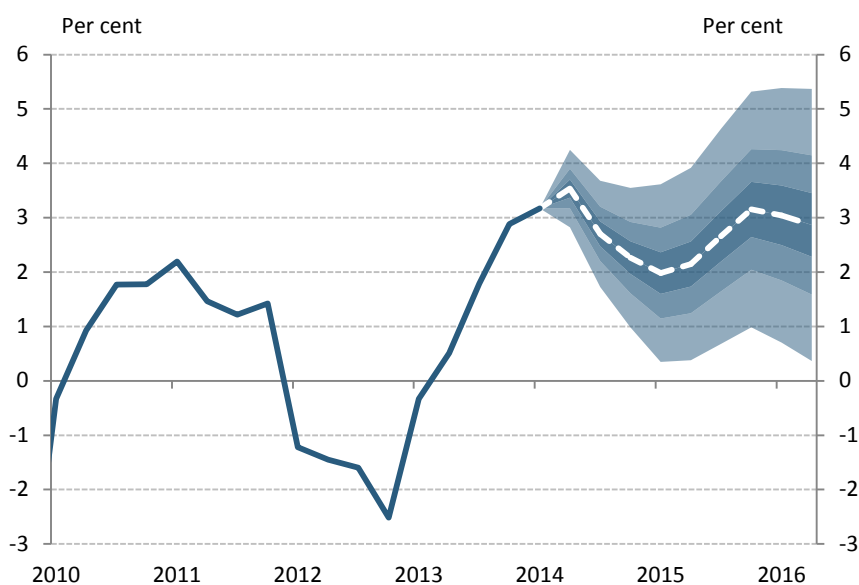
GDP projection fan chart
