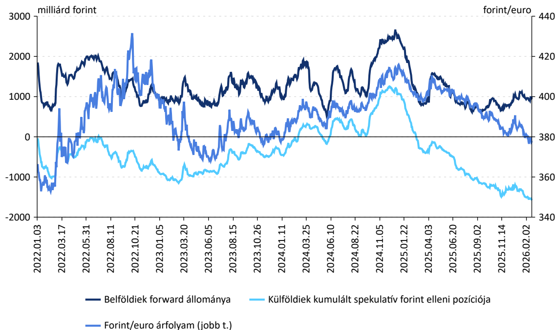
52. Belföldi és külföldi szereplők devizapiaci pozícionáltsága és a forint/euro árfolyam
