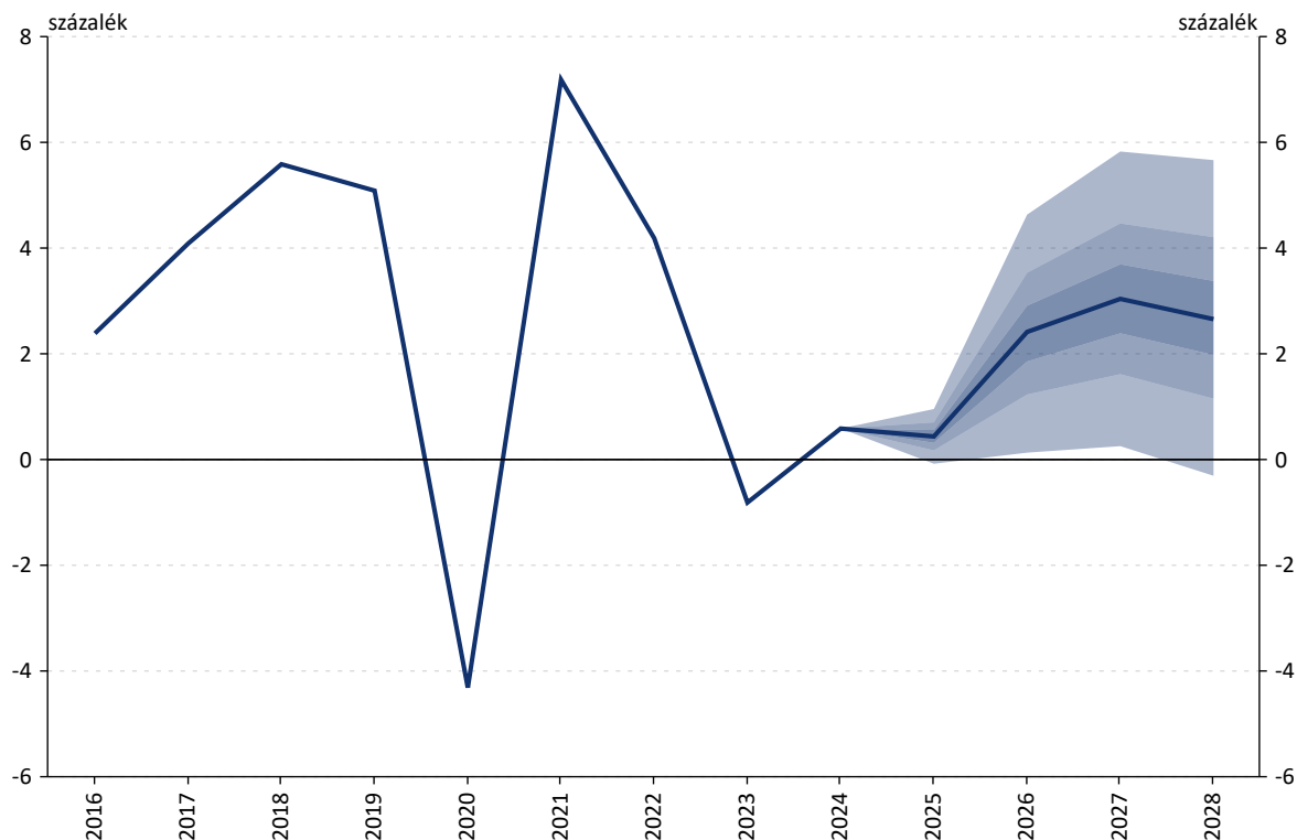
16. A GDP-előrejelzés legyezőábrája (2025. december)
