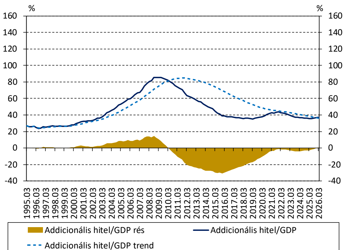
2. ábra: Az országspecifikus addicionális hitel/GDP rés alakulása
