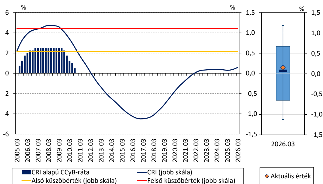
1. ábra: A ciklikus rendszerkockázati index (CRI) alakulása
