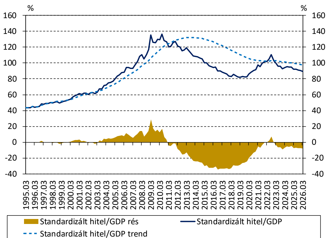
3. ábra: A standardizált hitel/GDP rész alakulása
