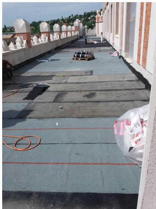
Legfelsőszint – ideiglenes vízszigetelése
