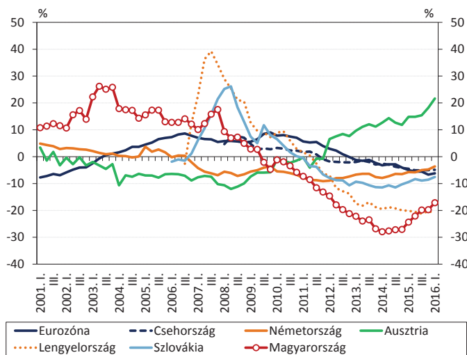
29. ábra: A nominális lakásárak/egy főre jutó nominális GDP százalékos eltérése a mutató hosszú távú átlagától
